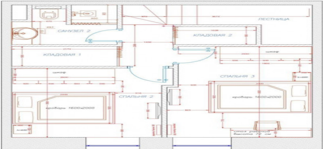
ТАУНХАУС 3 ЭТАЖ ЭКСПЛИКАЦИЯ
