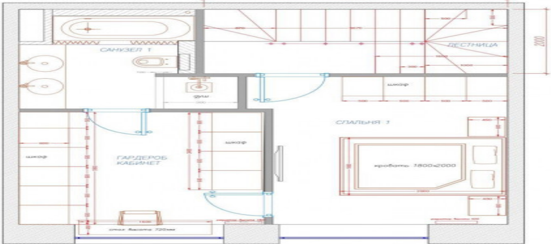
ТАУНХАУС 2 ЭТАЖ ЭКСПЛИКАЦИЯ
