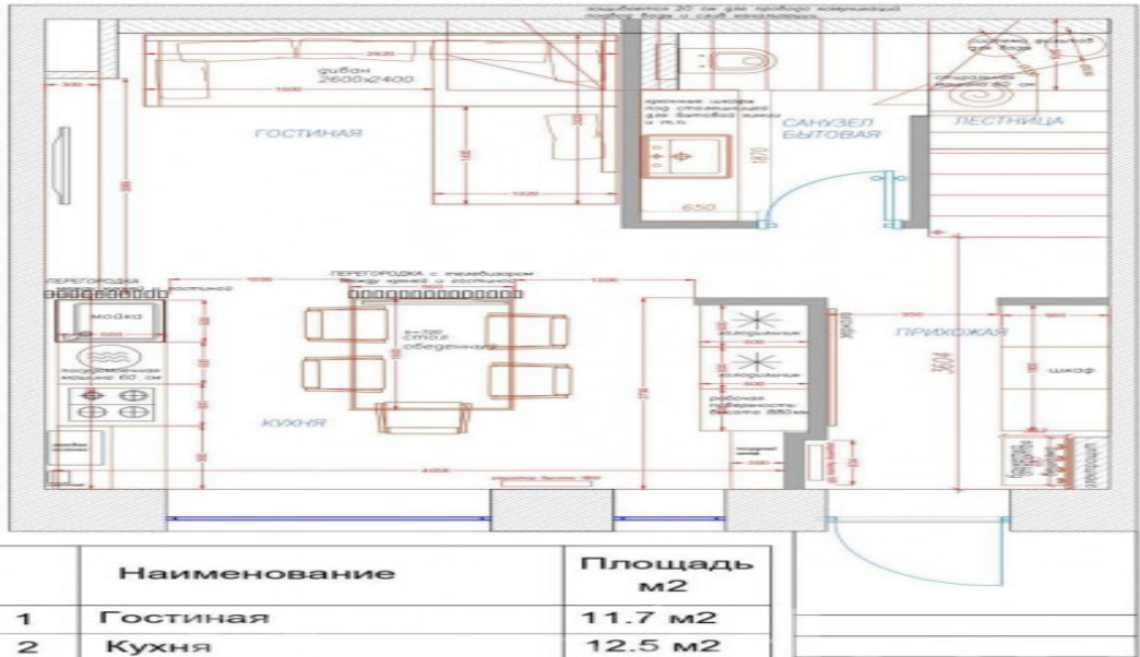
ТАУНХАУС 1 ЭТАЖ
