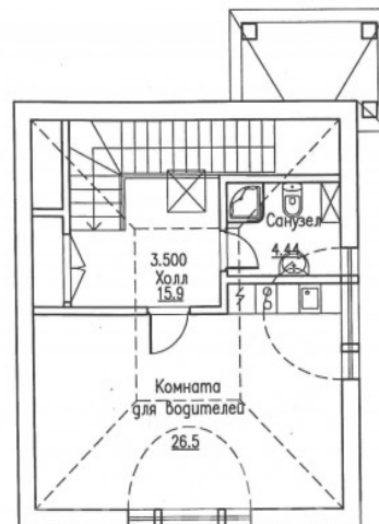
План мансардного этажа (М 1:100)
